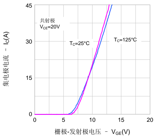
图3. 传输特性
