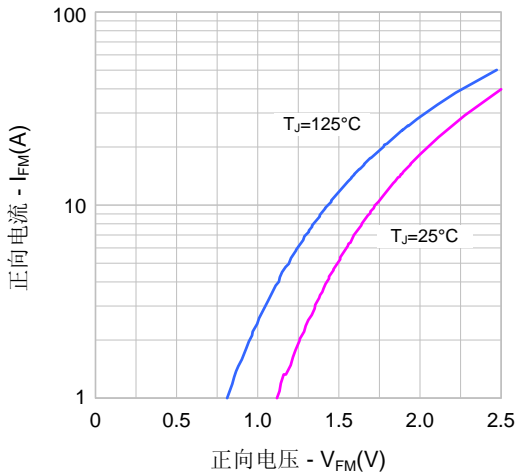
图15. 正向特性
